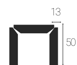
Kit WB4G 13x50mm Vista técnica
